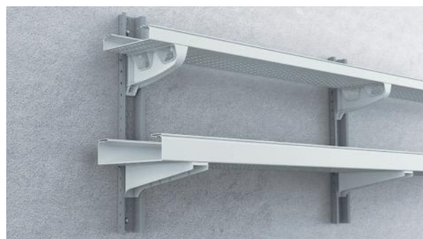
Perfil Ω perforado disponible en: · Acero galvanizado con pintura epoxy gris. · Acero inoxidable AISI 304 con pintura epoxy gris. Con soportes horizontales aislantes en U23X y U48X .
