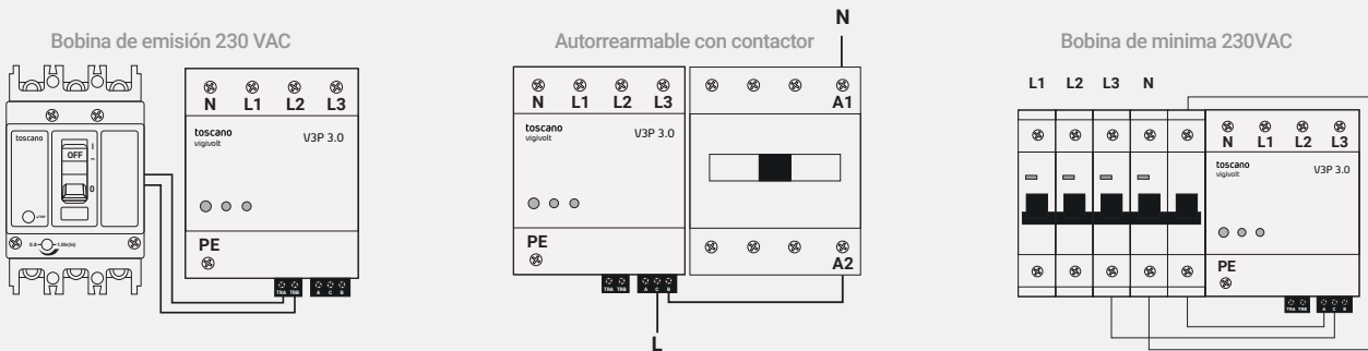
Esquema conexionado V3P3.0 / TRIO 3.0
