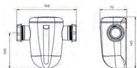
Dimensiones (mm)
