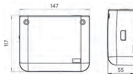
Dimensiones (mm)
