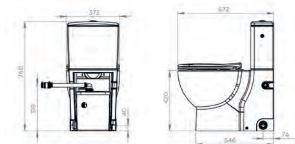
Dimensiones (mm)
