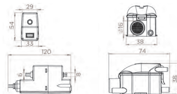
Dimensiones (mm)
