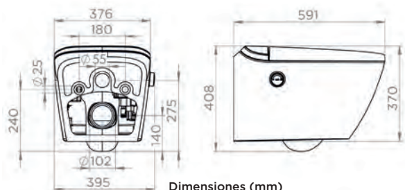
Dimensiones (mm)
