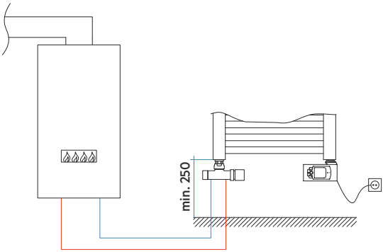
EJEMPLO DE FUNCIONAMIENTO MIXTO EN INSTALACIÓN MONOTUBO
