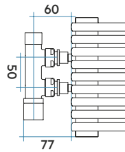
Conexión con manguitos y válvula toma 50 mm (Figura 13)
