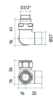
Vista frontal detentor
