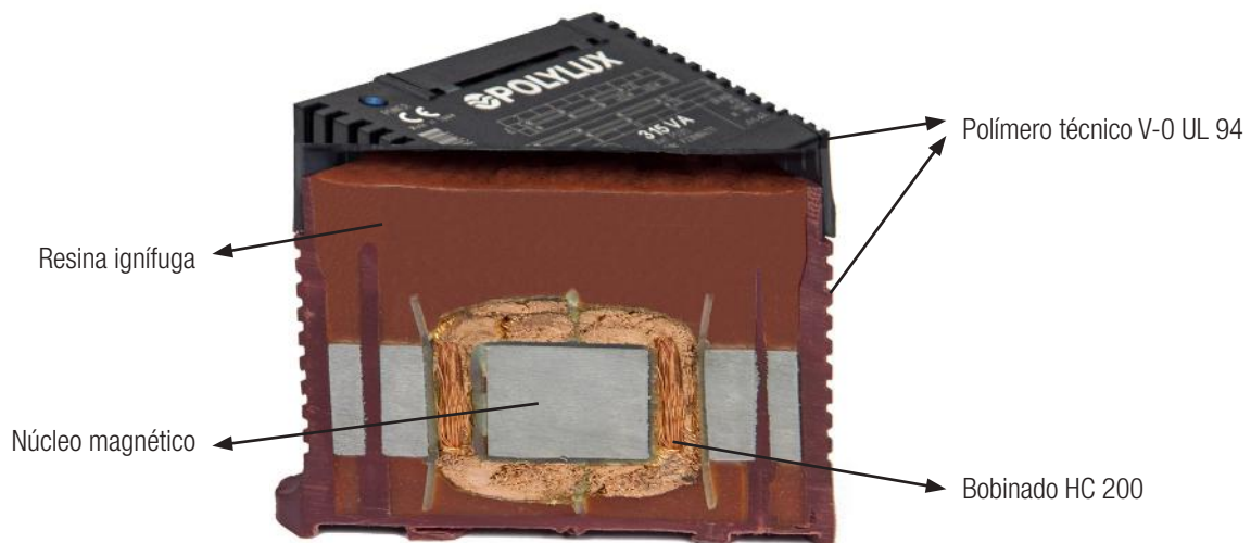
Transformador seccionado
