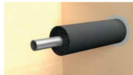
Tuberías combustibles hasta \varnothing 76 mm. (Tuberías de PP, PVC y multicapa)
